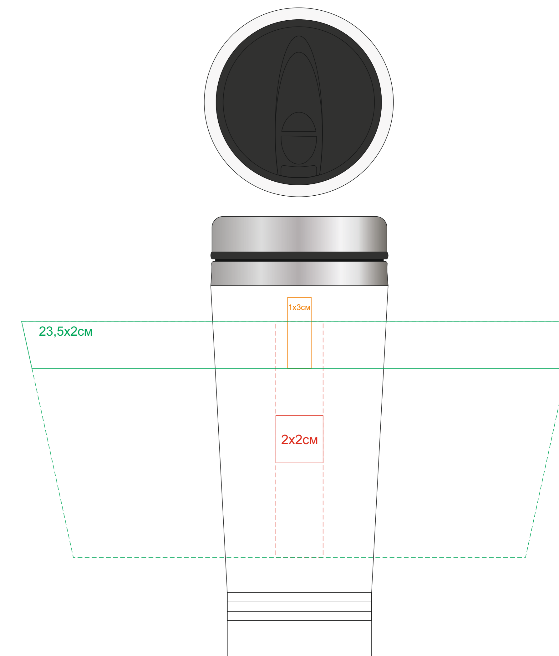
Питьевой клапан(лицо)
