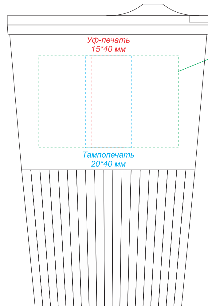
вид слева
